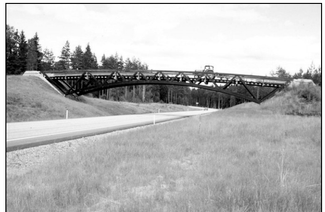
Skubbergsenga bru v/ Matrand - som er vernet
