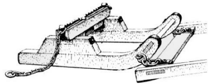
Stutting – brukt til lunning av tømmer. Tegning fra Skogbruksboka 4. Oslo 1960.
